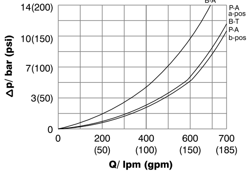
Spool Type 56
