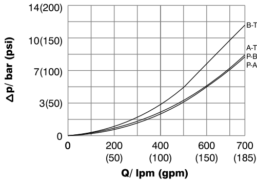
Spool Type 14
