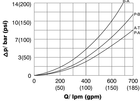
Spool Type 55
