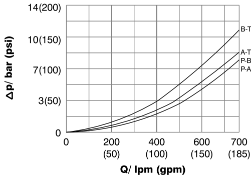
Spool Type 13
